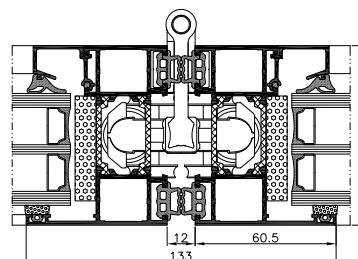
Assemblage de vantaux de porte, vue en coupe
