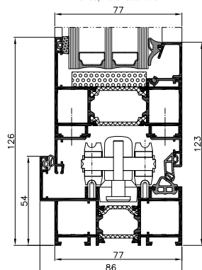
Porte, vue latérale
